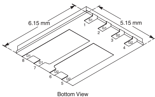
PowerPAK® SO-8
