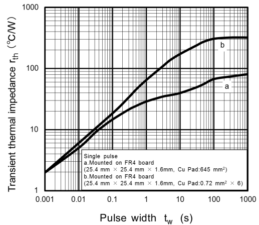
Fig. 7.12 r_{th} - t_w
