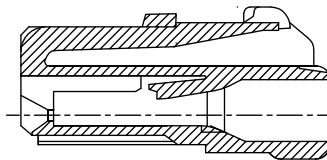
断面A-A SECT A-A
