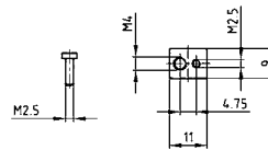
Mounting set for DIN EN 60603-2
