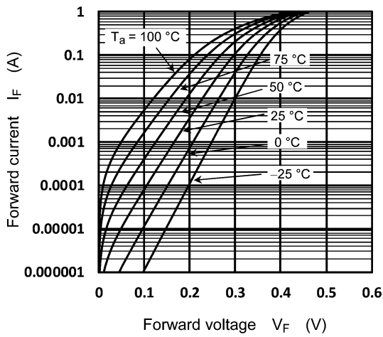
Fig. 9.1 I_F - V_F
