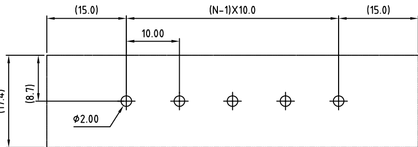
P.C.B LAYOUT
