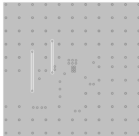
Bottom Layer
