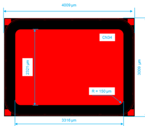
DIE OUTLINE
