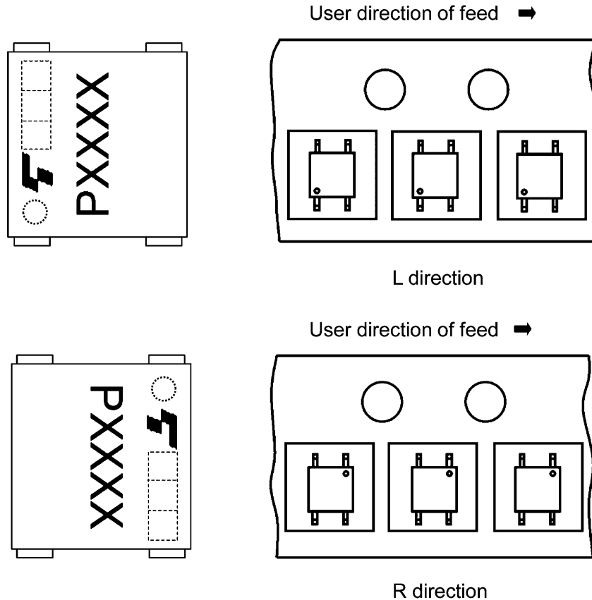
Fig. 16.3.1.1 Device Orientation
