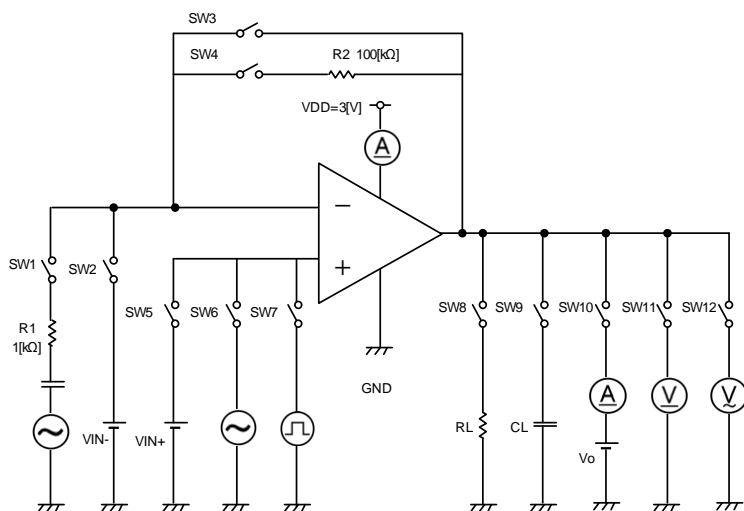
Fig. 95.. Test circuit2
