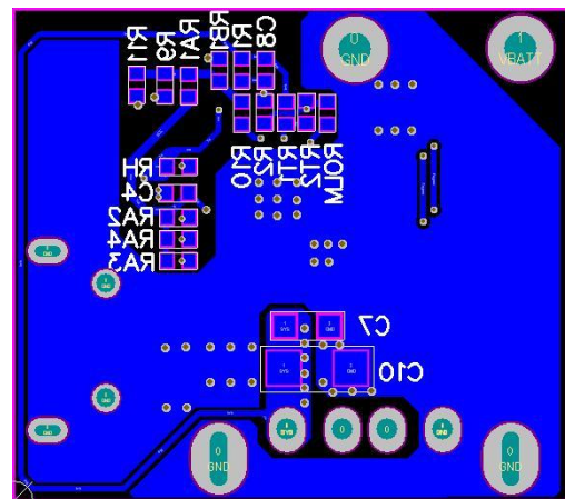
Bottom Layer
